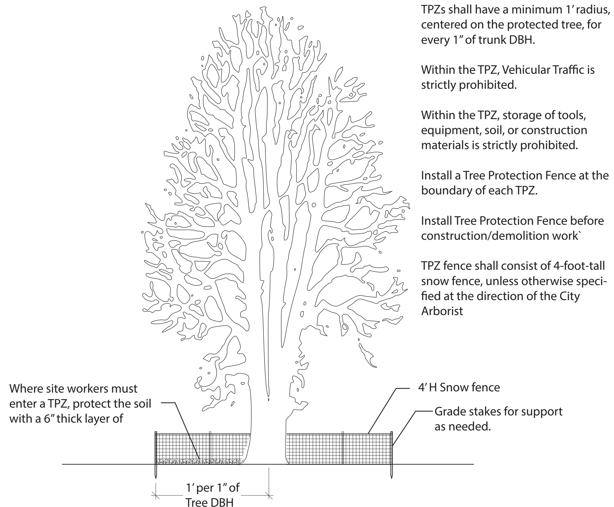
2 Tree Protection Zone (TPZ) Fence Detail (N.T.S.)
