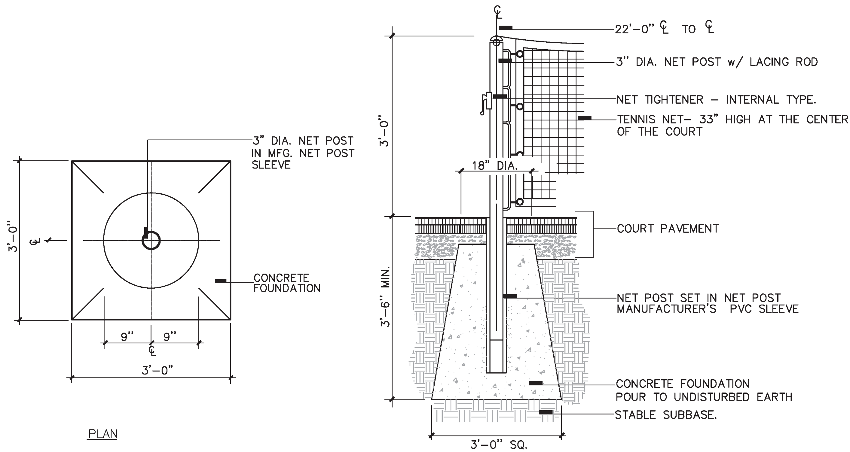
3 Net Post footing Detail (N.T.S.)
