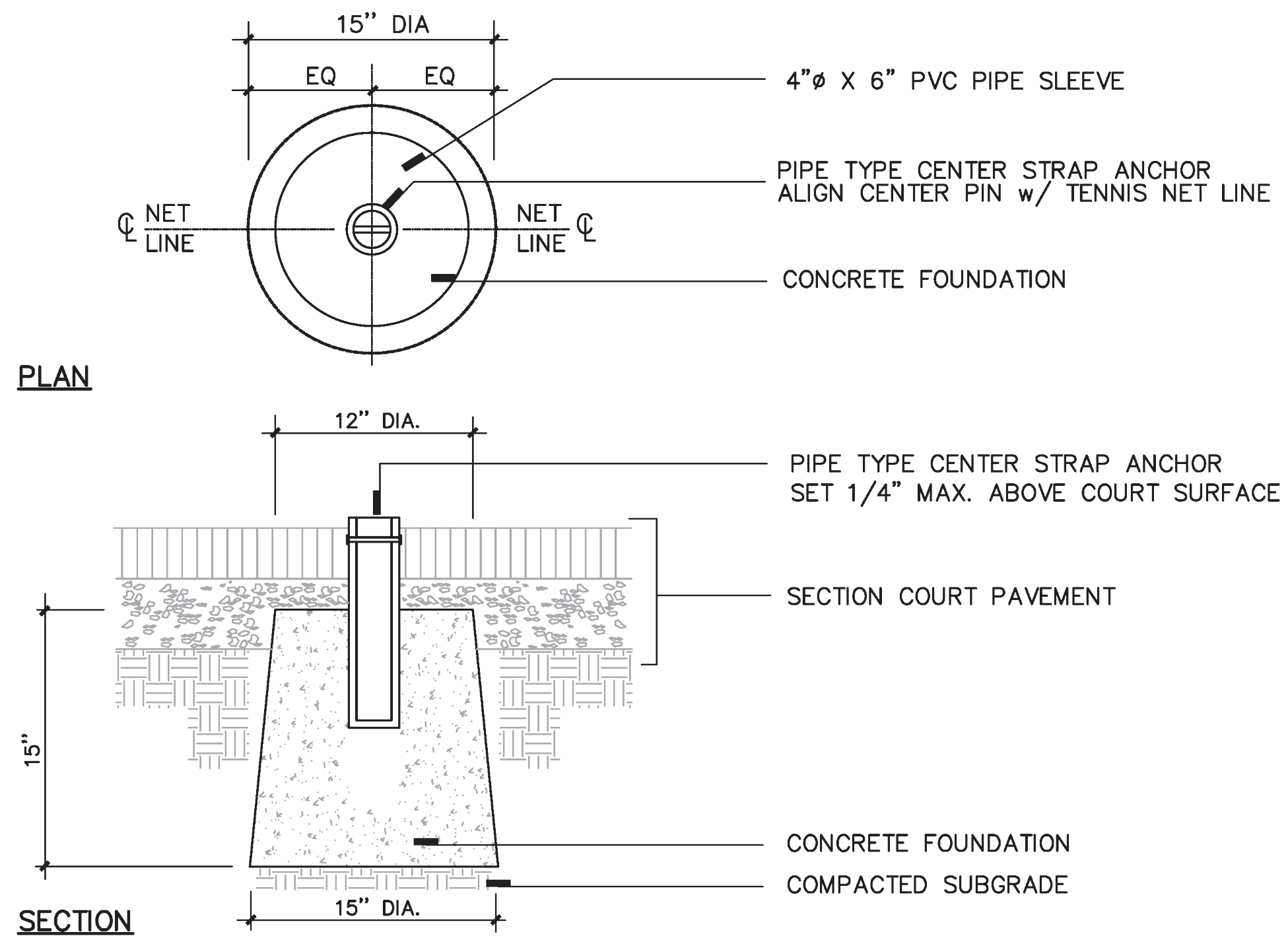
4 Center Strap Anchor Detail (N.T.S.)
